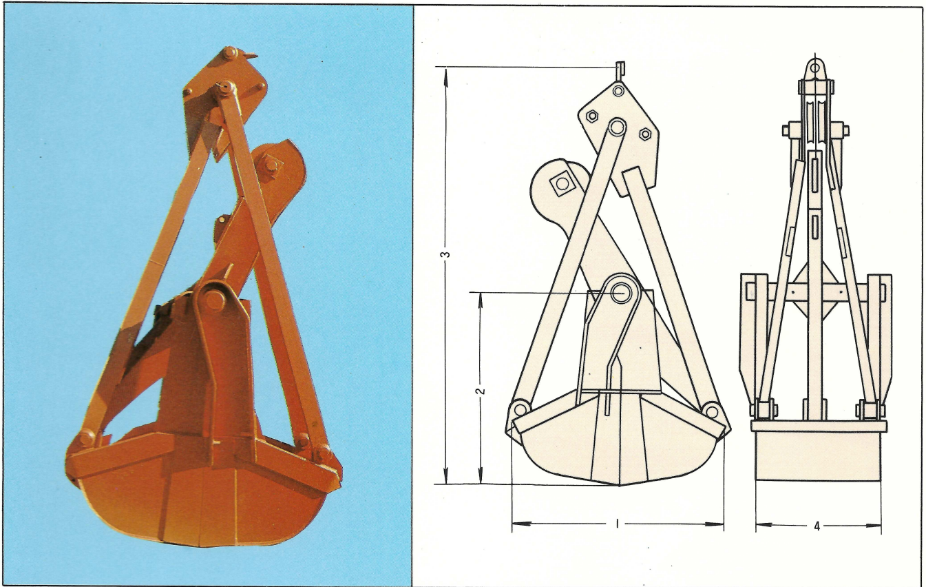
標準型ラッチアーム式バケット主要寸法表
