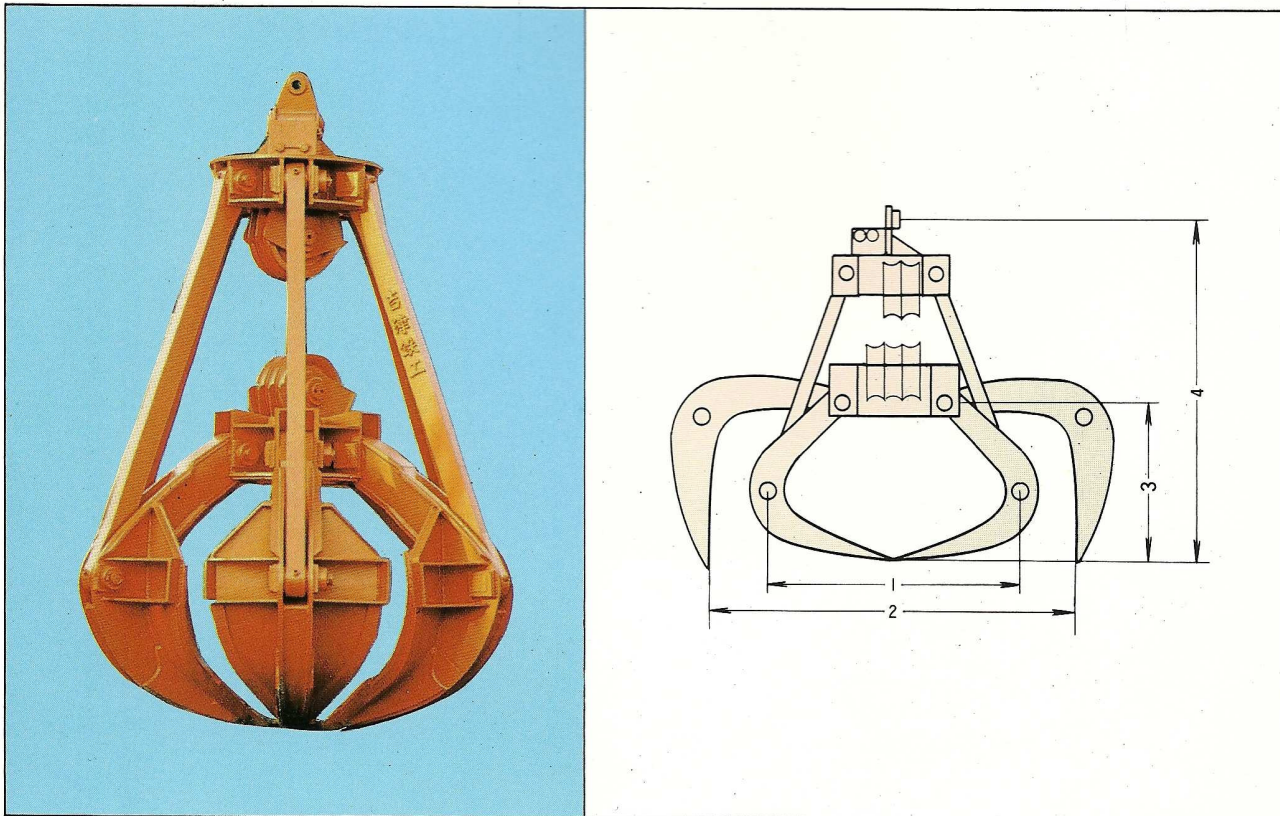
オレンジピール式バケット主要寸法表
